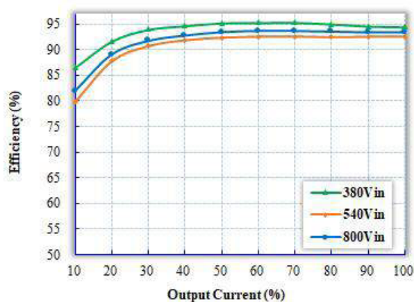
图(1): T_{case}=25^{\circ}\text{C} , 分别在最小输入电压, 额定输入电压, 最大输入电压时, 不同负载时的效率曲线。
