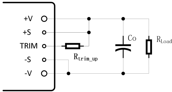
图(16)输出电压上调 TRIM 电阻接法示意图
