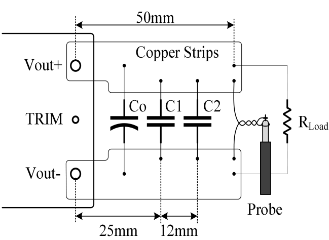
图(15)输出纹波与噪声测试示意图
