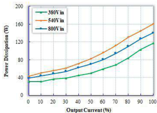
图(2): T_{case}=25^{\circ}\text{C} , 分别在最小输入电压, 额定输入电压, 最大输入电压时, 不同负载时的损耗。
