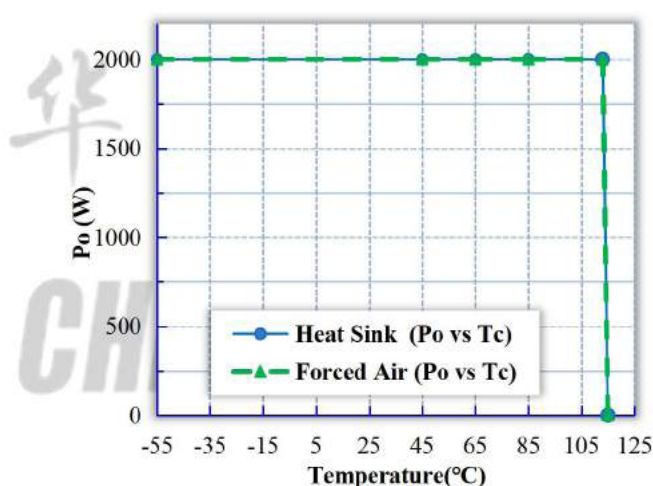
图(4): 额定输入时的温度降额曲线
