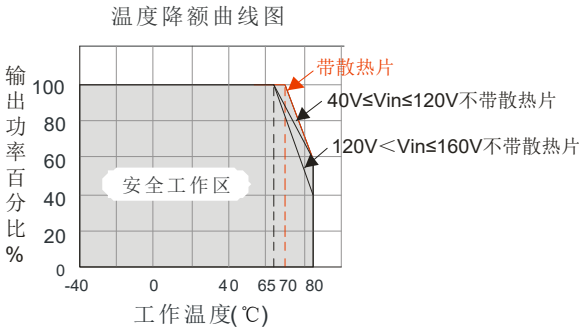
CFDA20-110S03GC工作温度曲线
