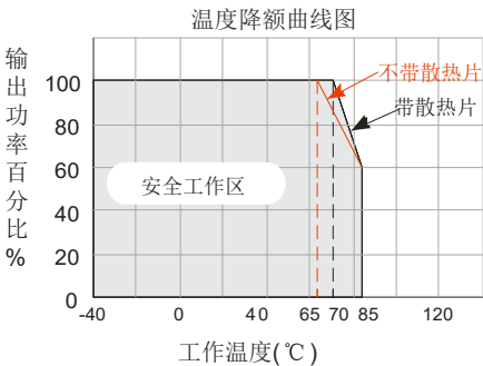
CFDA20-110S12/15/24/28工作温度曲线
