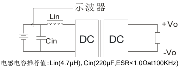
电感电容推荐值: Lin(4.7μH), Cin(220μF, ESR<1.0Ωat100KHz)
