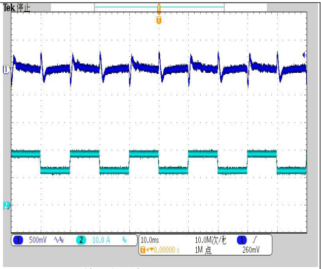
CH1:输出电压波形(500mV/div) CH2:输出电流波形(10.0A/div) 图(12)输出纹波电压波形图
