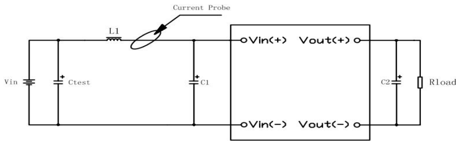
图(15)输入反射纹波电流测试示意图
