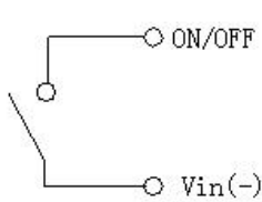
图(14a) 开关控制方式
