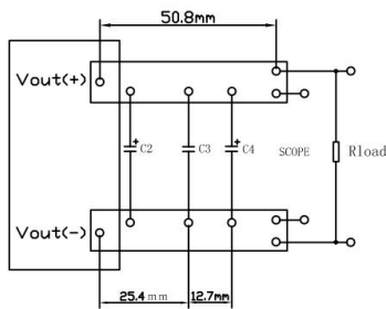
图(16)输出纹波与噪声测试示意图
