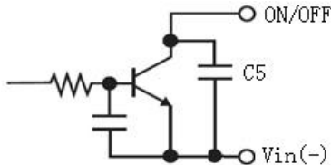
图(14b) 晶体管控制方式
