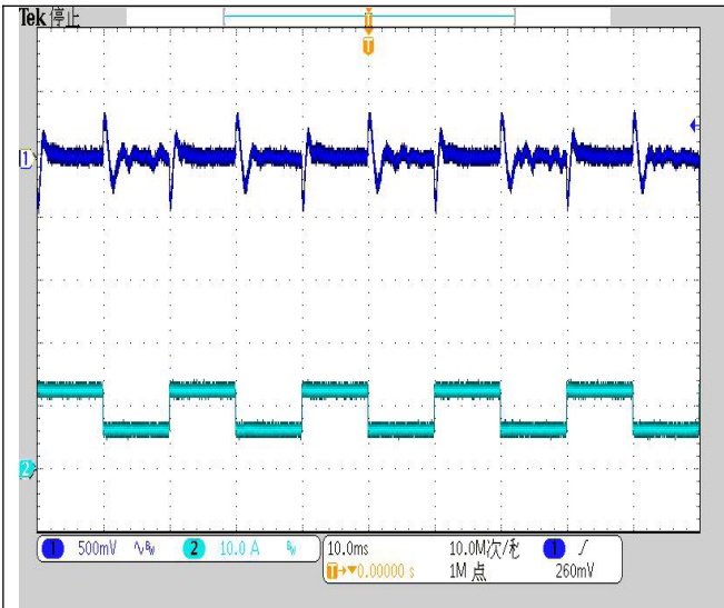
CH1:输出电压波形(500mV/div) CH2:输出电流波形(10.0A/div) 图(11)输入反射纹波电流波形图
