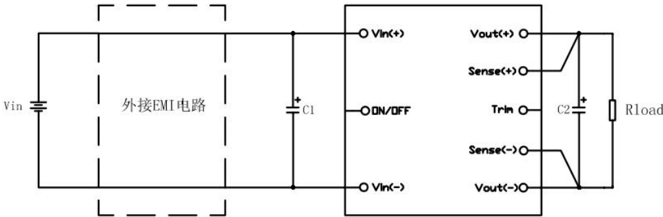
图(13)典型应用电路
