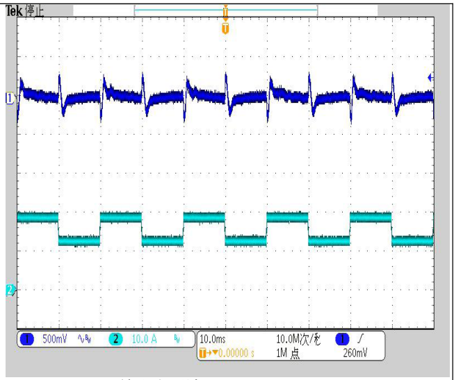
CH1:输出电压波形(500mV/div) CH2:输出电流波形(10.0A/div) 图(12)输出纹波电压波形图
