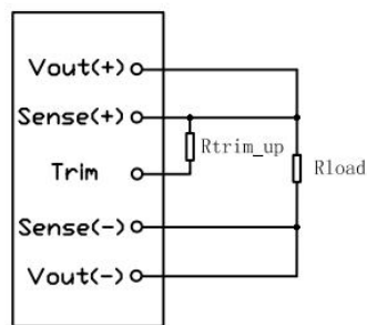
图(17)输出电压上调示意图
