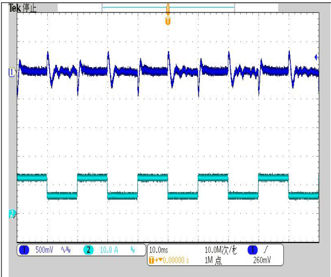
CH1:输出电压波形(500mV/div) CH2:输出电流波形(10.0A/div) 图(11)输入反射纹波电流波形图
