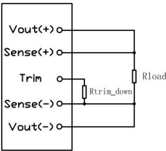
图(18)输出电压下调示意图
