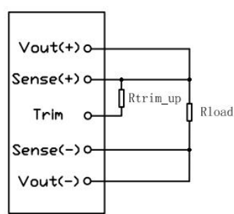
图(17)输出电压上调示意图
