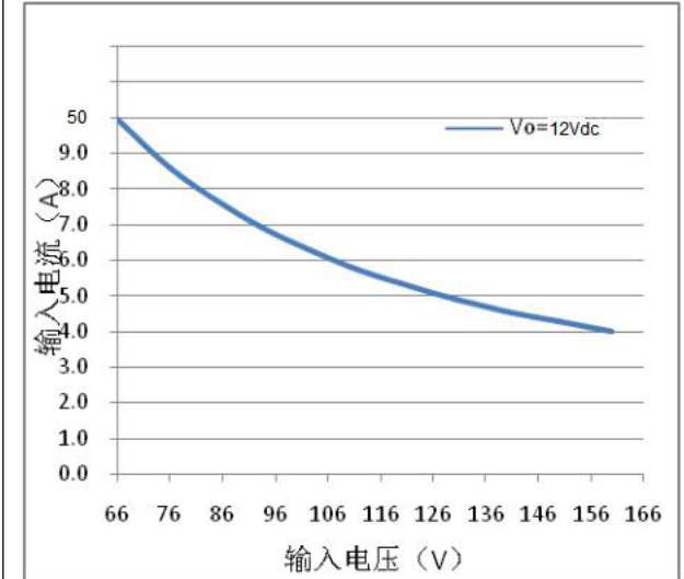
图(3)输入特性曲线图(Tc=25℃)
