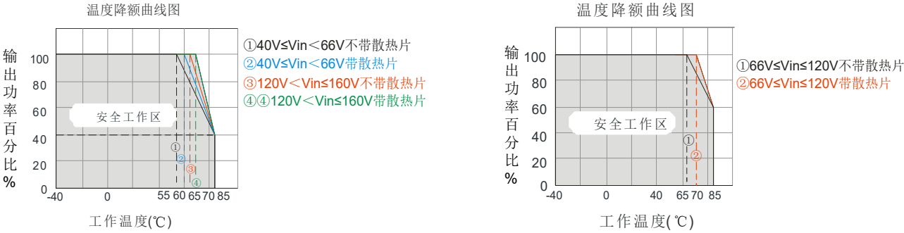
CFDA20-110S05GC工作温度曲线
