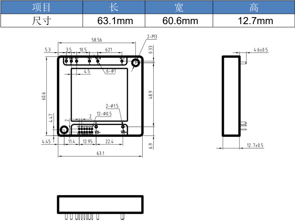
模块结构图
