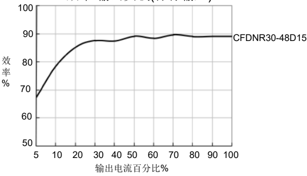
效率/输出负载(标称输入)
