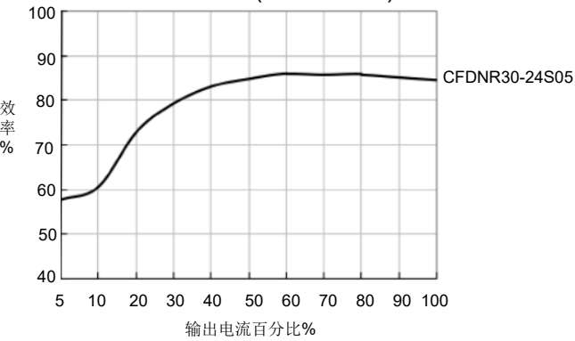
效率/输出负载(Vin=24VDC)
