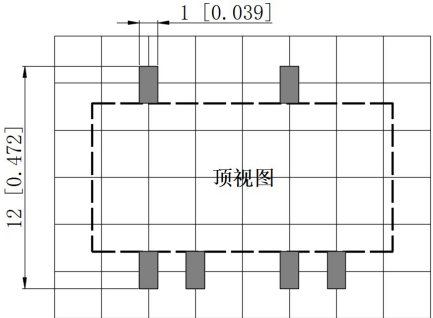
注: 栅格距离尺寸为 2.54*2.54mm
