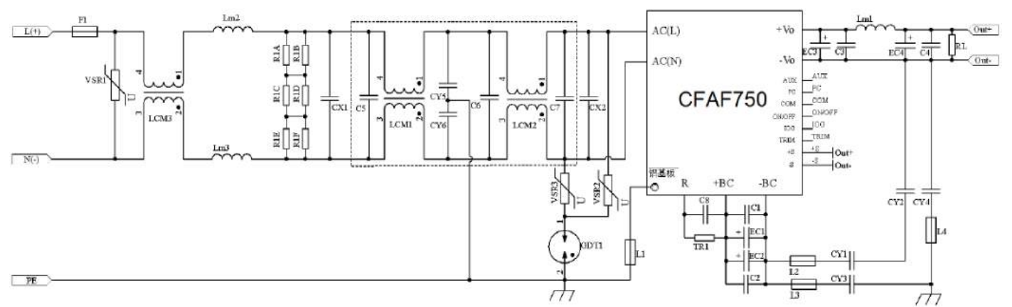
图2: 推荐电路2
