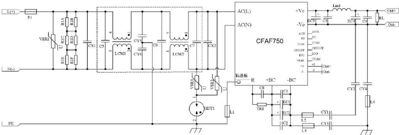
图1:推荐电路1
