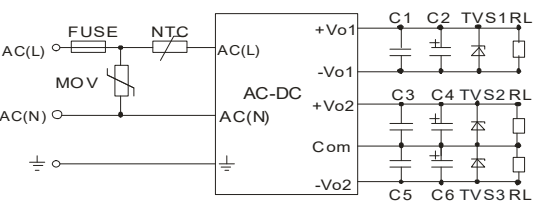
图3: 三路典型应用电路
