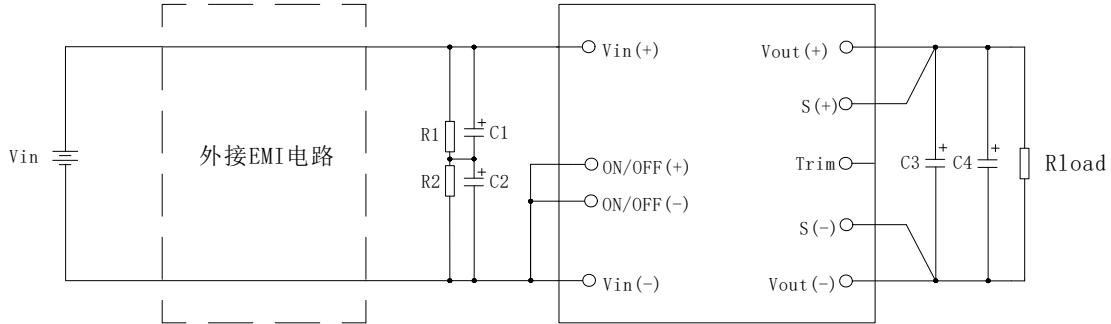
图5 典型应用电路
