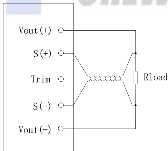
图11 输出电压远端补偿电路
