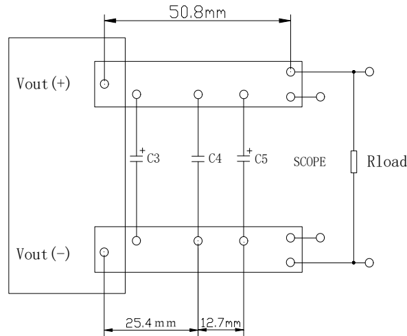
图8 输出纹波与噪声测试示意图
