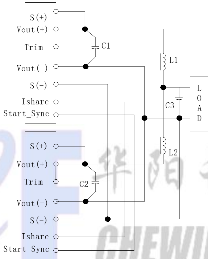
图12 多路输出并联示意图
