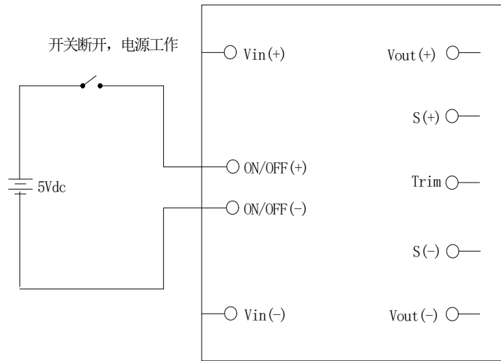
图 6 遥控端控制方式示意图
