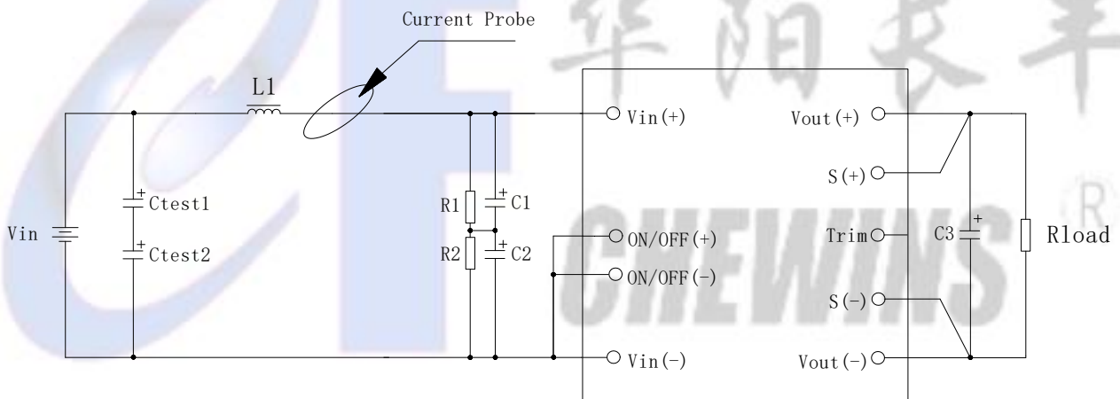
图7 反射电流测试示意图
