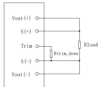
图10 输出电压下调示意图
