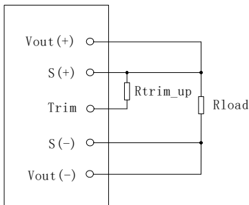
图9 输出电压上调示意图
