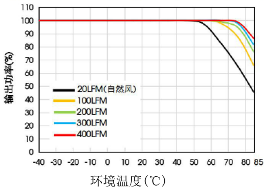
CFDQR100-48S24温度降额曲线( V_{in}=24V )
