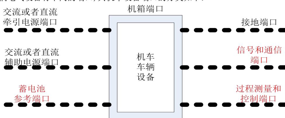
图 3. 机车电气设备接口
