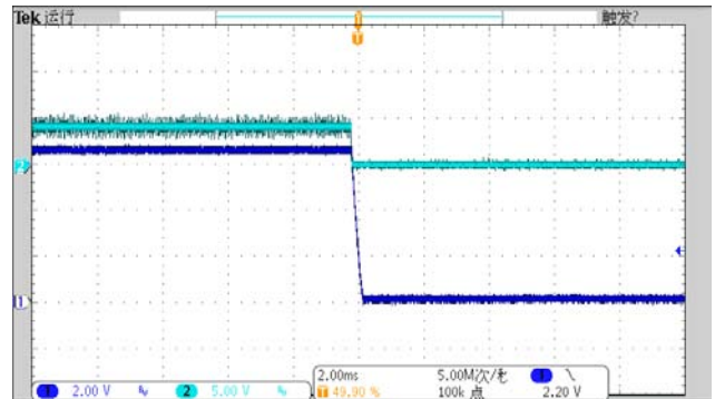
图（8）ON/OFF关机波形图
