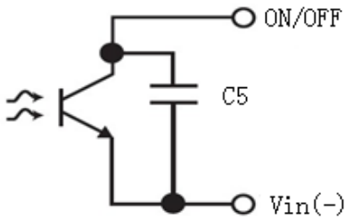
图 (14c) 隔离控制方式
