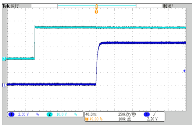
图（5）电源开机波形图
