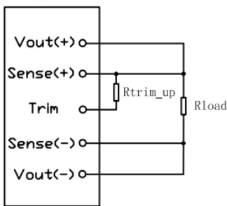
图（17）输出电压上调示意图
