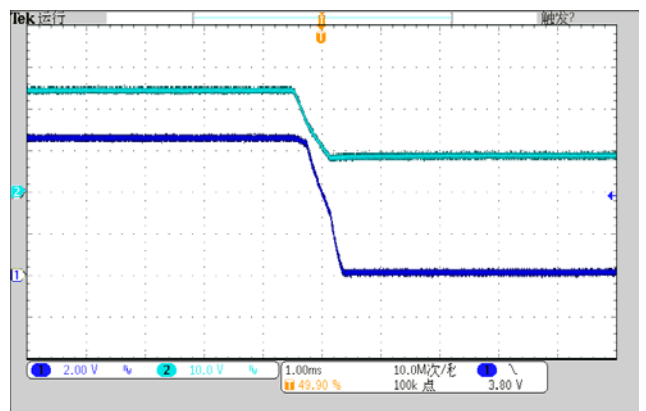
图（6）电源关机波形图
