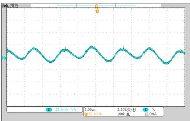
图（11）输入反射纹波电流波形图
