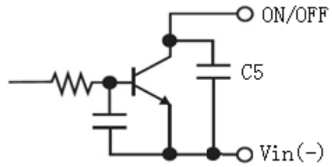
图 (14b) 晶体管控制方式
