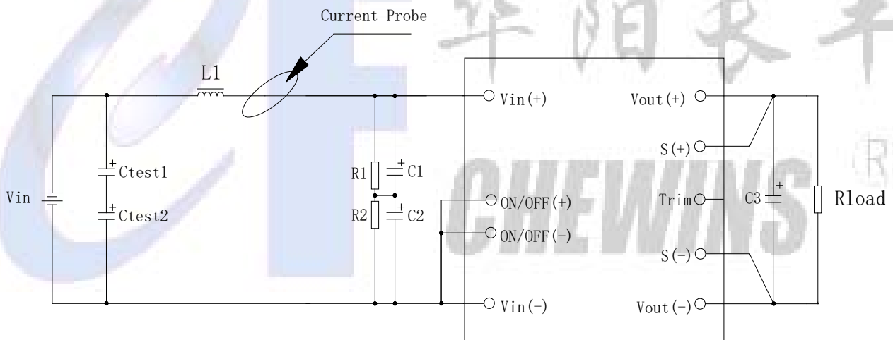
图（15）反射电流测试示意图
