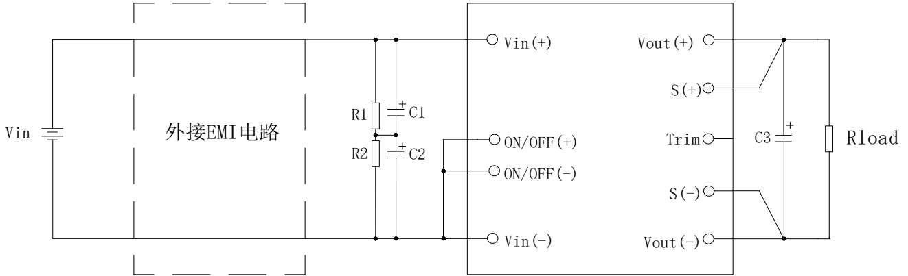
图（13）典型应用电路
