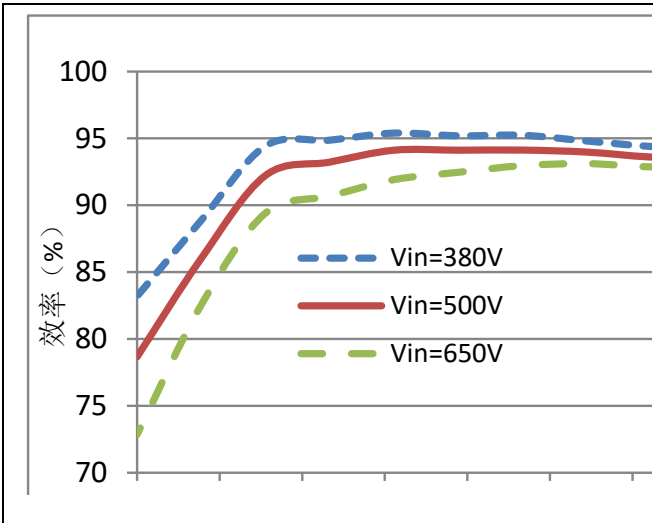
图 (3) 输入特性曲线图
