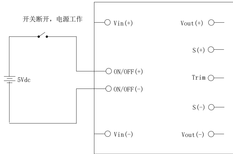
图（14）遥控端控制方式示意图
