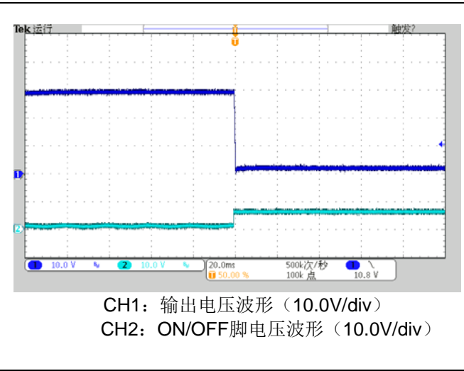
图 (10) 50%-75%-50% (2.5A/μs) 动态波形图
