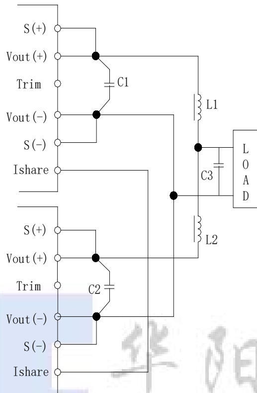
图 (20) 多路输出并联示意图
