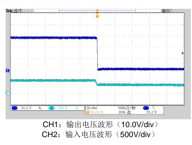
图 (8) ON/OFF 关机波形图
