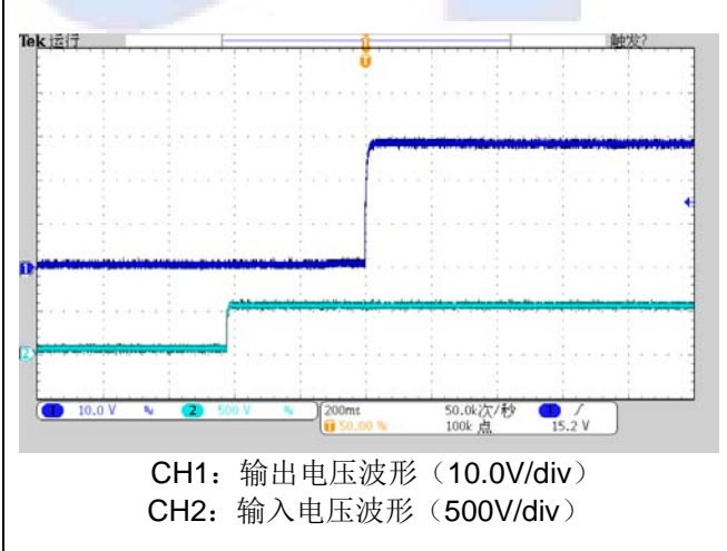
图 (7) ON/OFF 开机波形图
