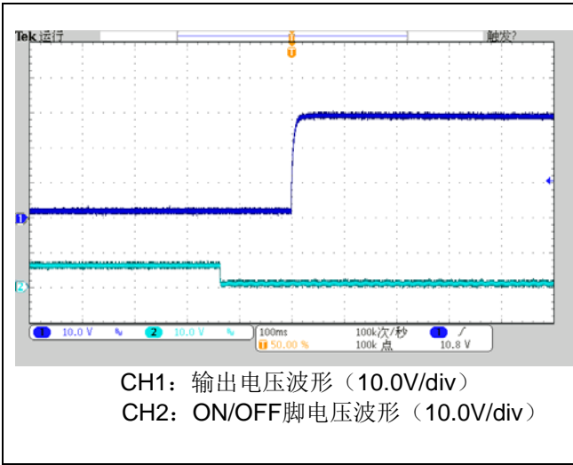
图 (9) 25%-50%-25% (2.5A/μs) 动态波形图
