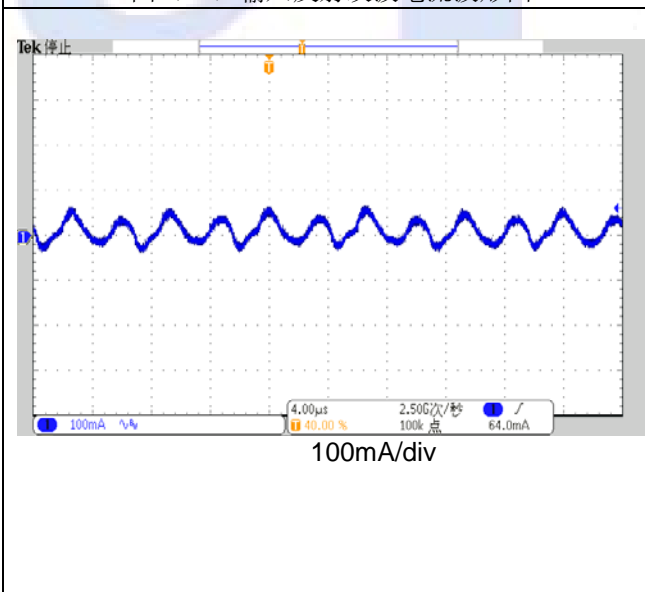
图 (11) 输入反射纹波电流波形图
