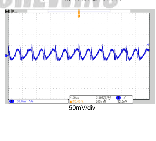
图 (12) 输出纹波电压波形图
