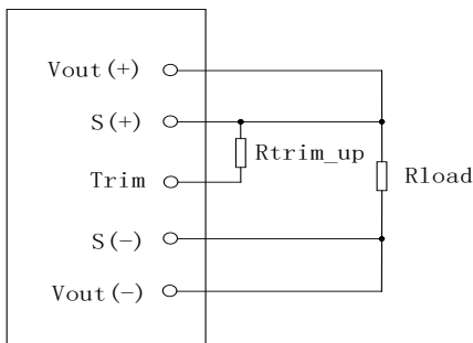
图（17）输出电压上调示意图
