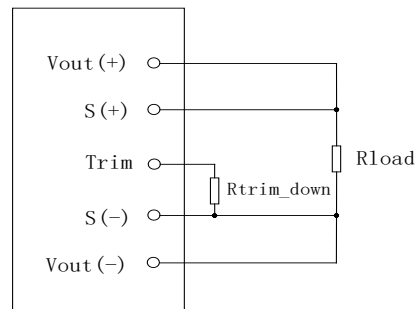
图（18）输出电压下调示意图
