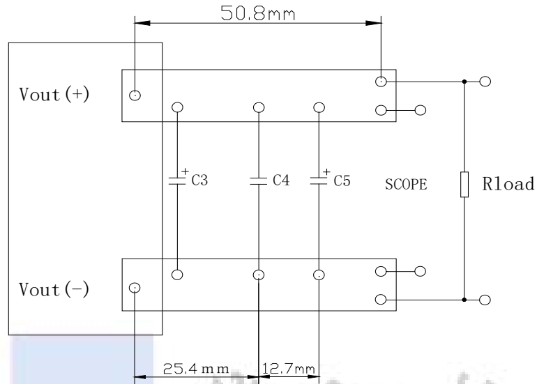
图（16）输出纹波与噪声测试示意图
