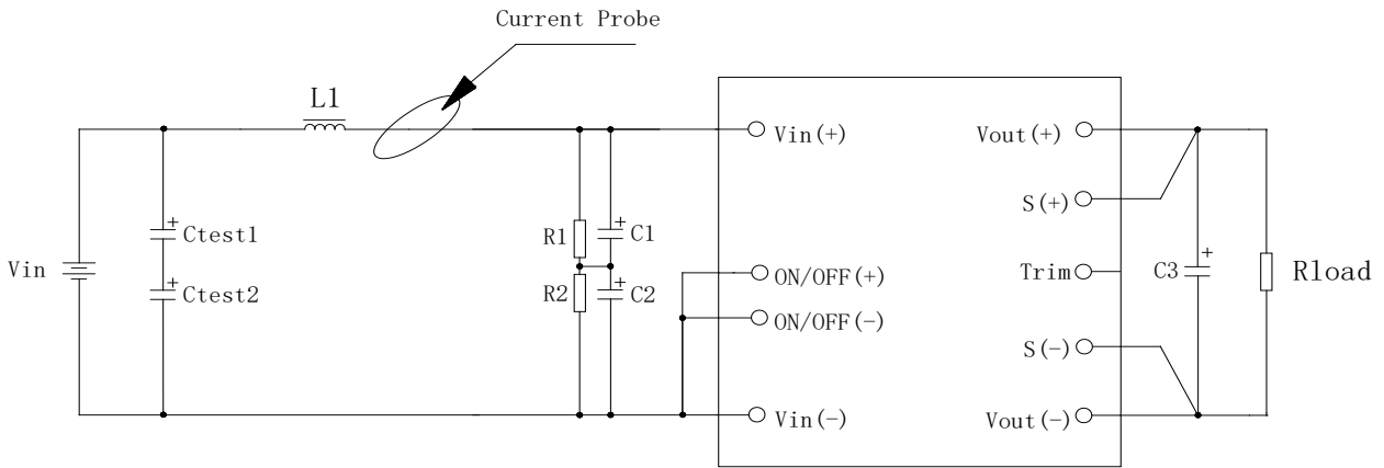
图 (15) 反射电流测试示意图
