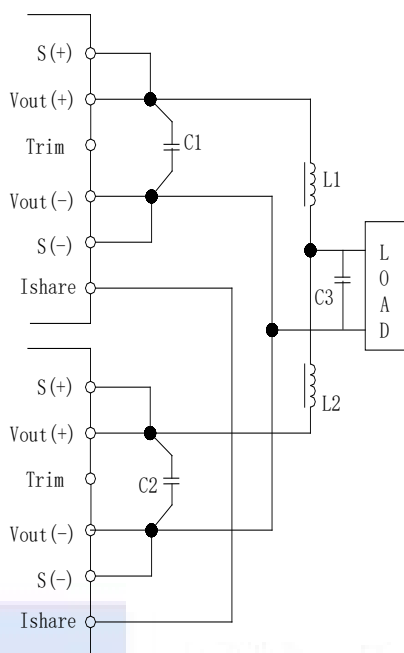
图（20）多路输出并联示意图（ C1=C2 \geq 560\mu , C3 \geq 1000\mu , L1=L2 > 1\mu H ）
