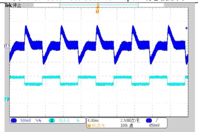
图 (10) 50%-75%-50% (0.1A/μs) 动态波形图
