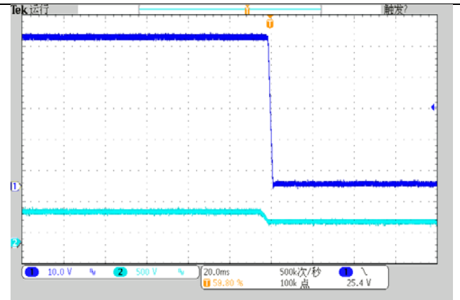
CH1: 输出电压波形 (10.0V/div) CH2: 输入电压波形 (500V/div)
