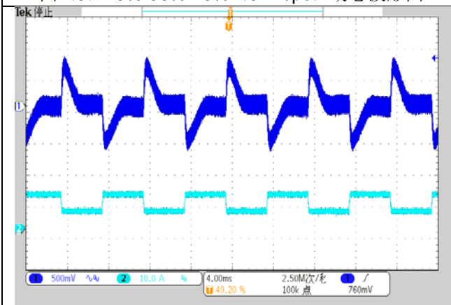
图 (9) 25%-50%-25% (0.1A/μs) 动态波形图
