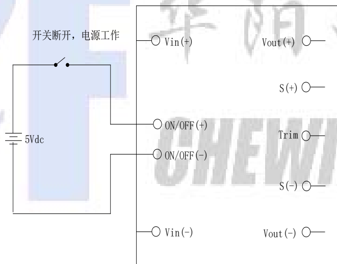
图（14）遥控端控制方式示意图
