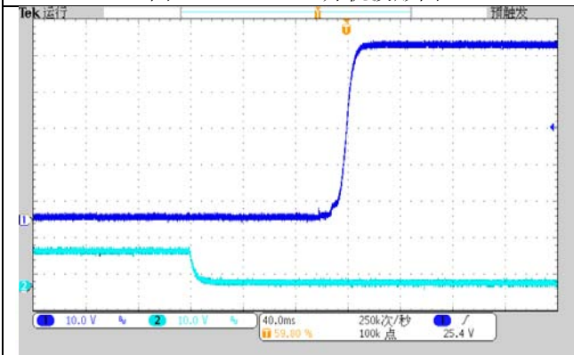
CH1: 输出电压波形 (10.0V/div) CH2: ON/OFF 脚电压波形 (10.0V/div)
