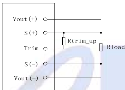
图 (17) 输出电压上调示意图
