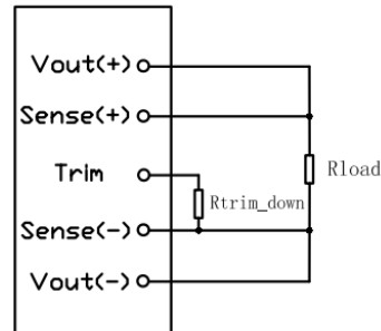
图（18）输出电压下调示意图
