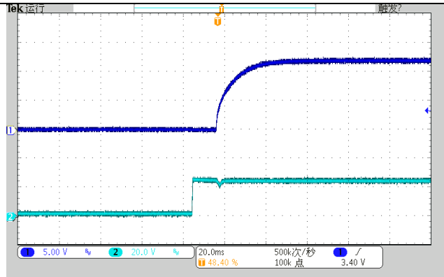
图（5）电源开机波形图
