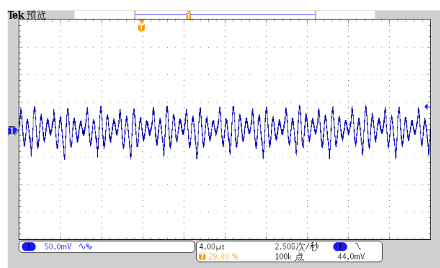
图（12）输出纹波电压波形图
