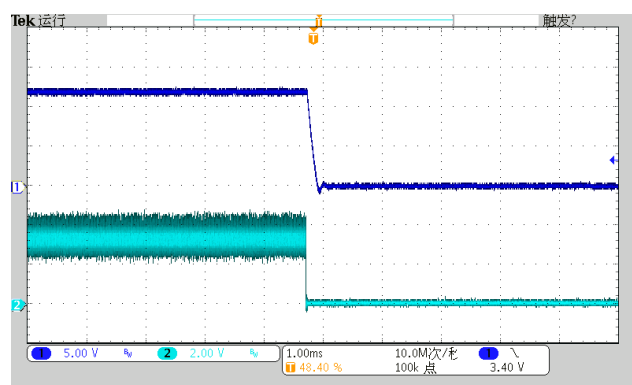
图（8）ON/OFF关机波形图
